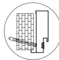
montážny otvor kotva vo falci zárubne
