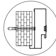
montážny otvor kotva v strede profilu zárubne
