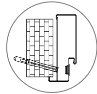
montážny otvor kotva vo falci zárubne
