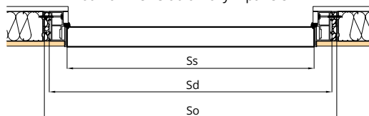
DVEŘE HARMONY INVEST (OTEVÍRÁNÍ VEN) ODZ
