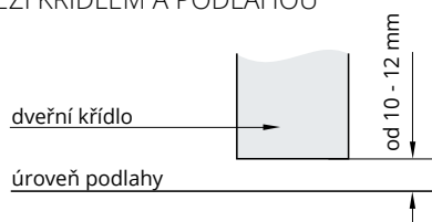
SVĚTLOST MEZI KŘÍDLEM A PODLAHOU
