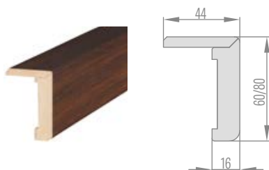
ŠTANDARDNÝ UHOLNÍK PRE NASTAVITEĽNÉ ZÁRUBNE
