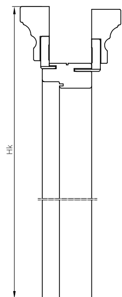
Sk – šířka po vnější straně korunky Hk – výška po vnější straně korunky
